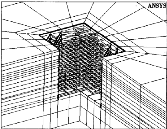
图 2 单元网格及支撑
