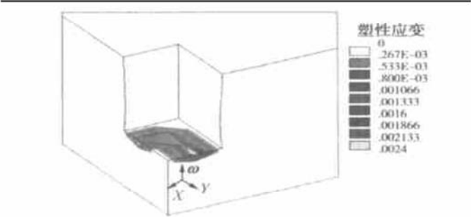
图 5 土体塑性区分布
