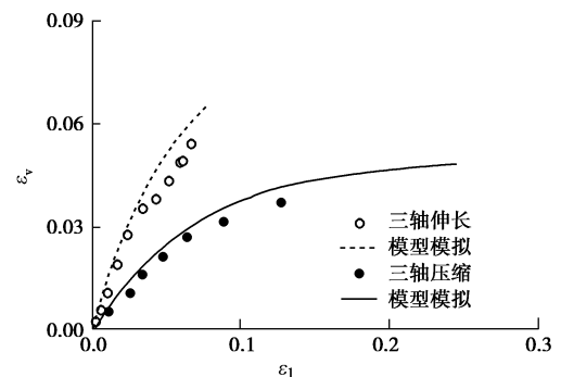
(c) 第一主应变与体变的关系
