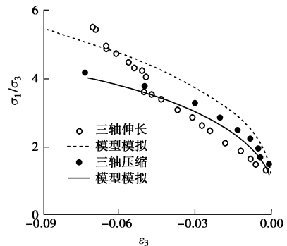
(b) 第三主应变与应力比的关系
