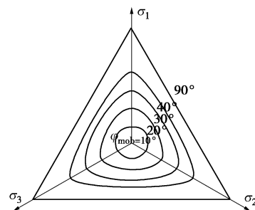
图1 \pi 平面上SMP准则的形状
