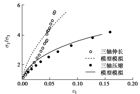
(a) 第一主应变与应力比的关系
