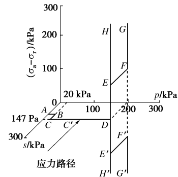
(a) 三轴试验中 ( p_{\text{net}}=196 \text{ kPa} ) 的应力路径
